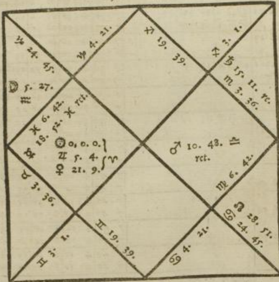
Figura cœli Verna, Die 9. Martij, hor: à merid: 17. min: 15.
