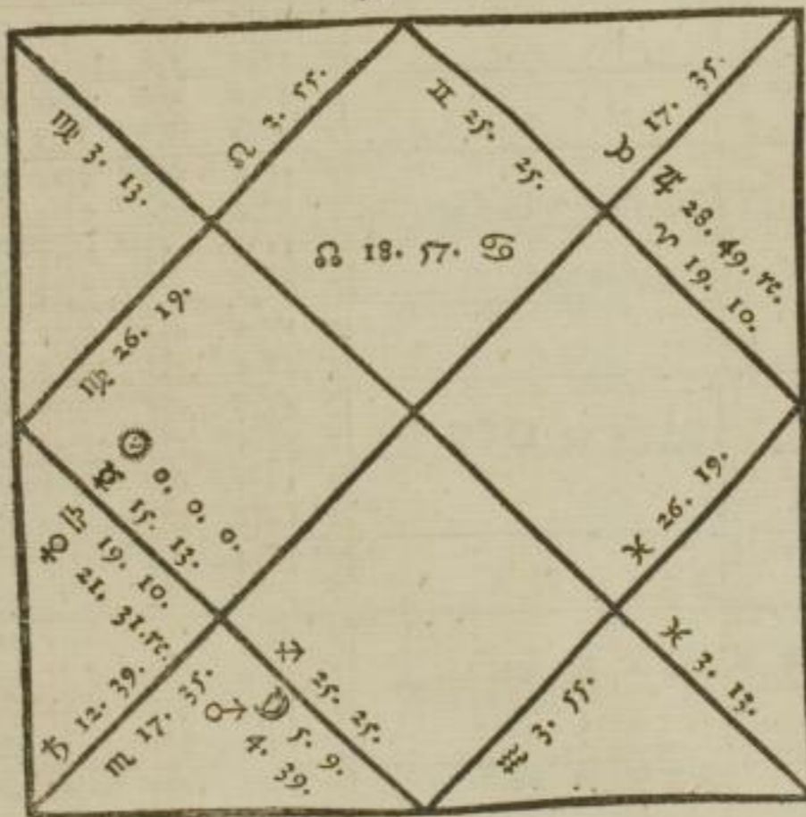
Figura cœli Autumnalis Die 12. Septembris, hor: à merid: 17. minut: 40.
