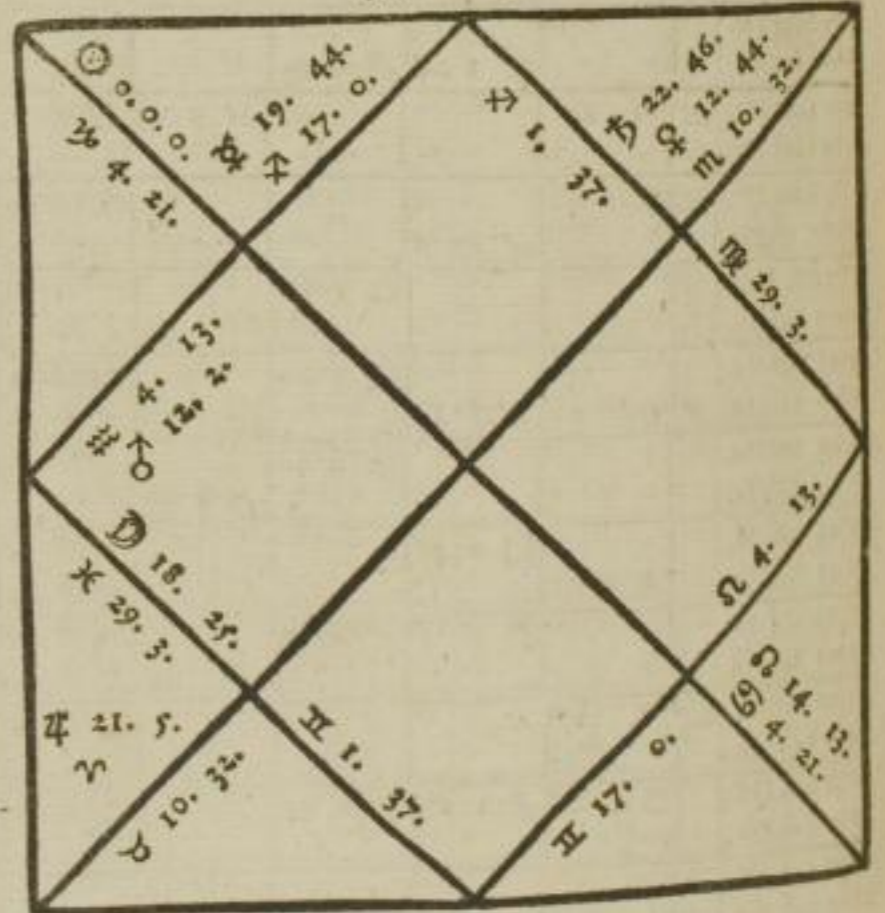
Figura cœli Hiemalis, Die 10. Decembris, hor: à merid: 21. minut: 58.
