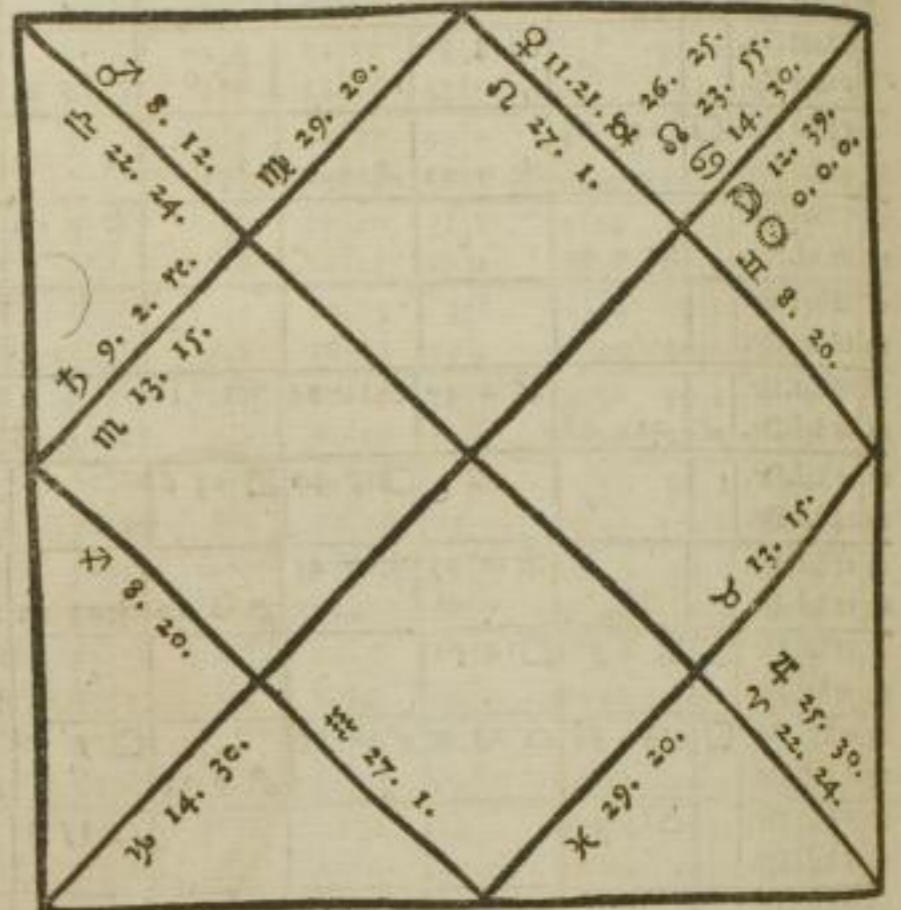
Figura cœli Æstiuæ, Die 11. Iunij, Hor: à merid: 3. min: 57.
