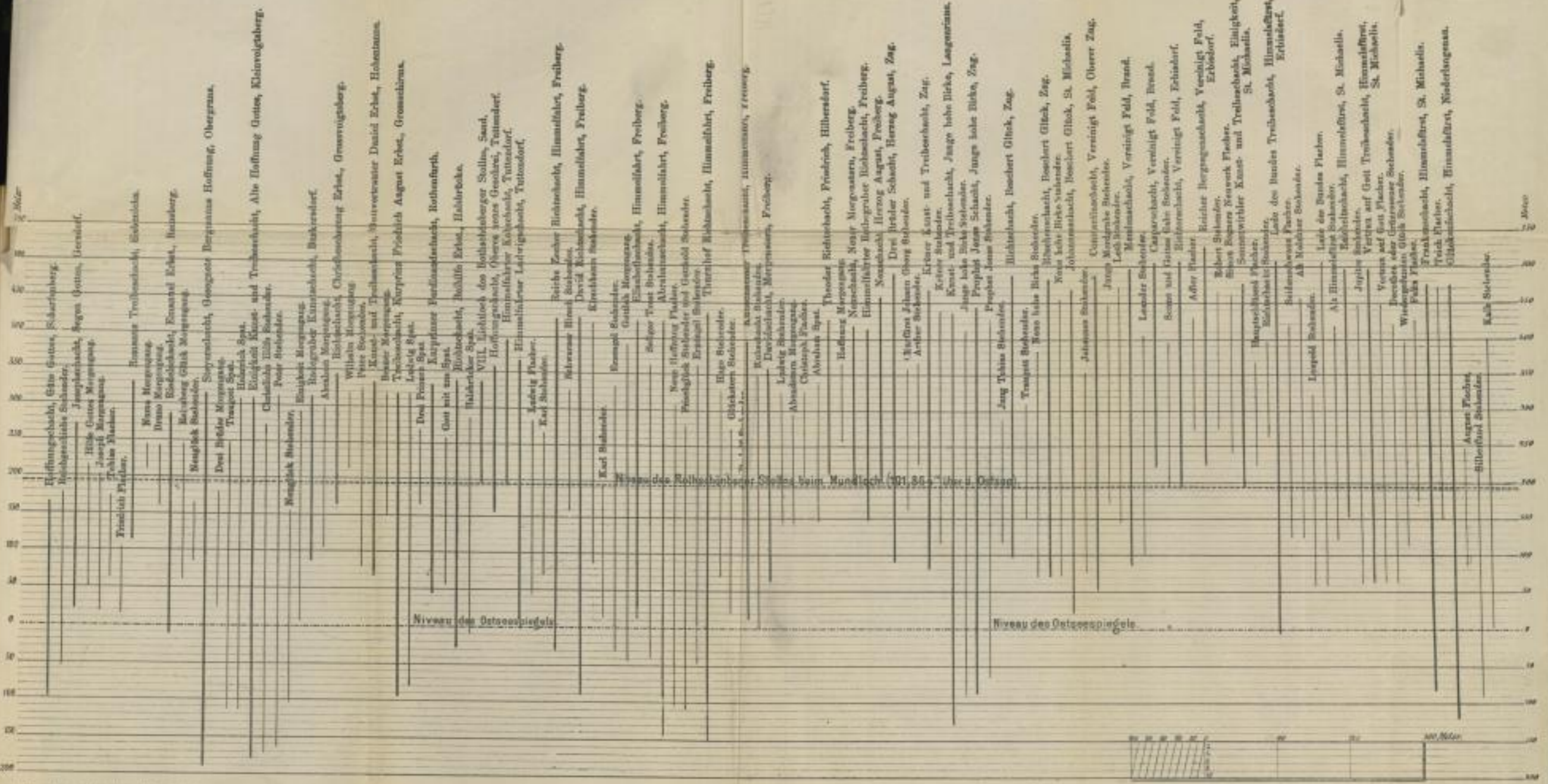
Graphische Darstellung der mit den Hauptschächten und den Abbauen auf den verschiedenen Erzgängen des Freiburger Reviers erreichten Seigerteufen unter Bezugnahme auf das Niveau des Ostseespiegels.
