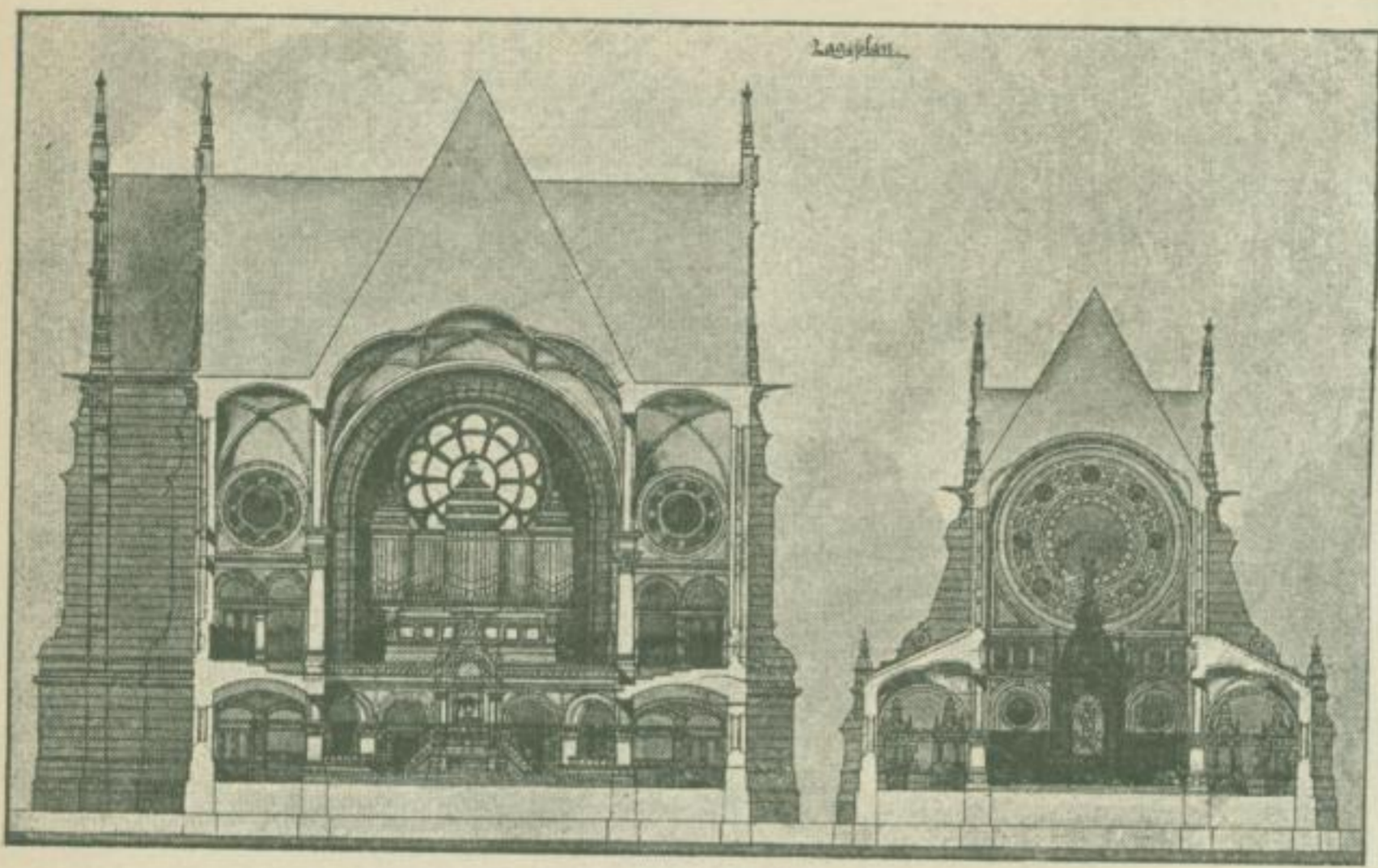
Querschnitt durch die evangel. Kirche.
