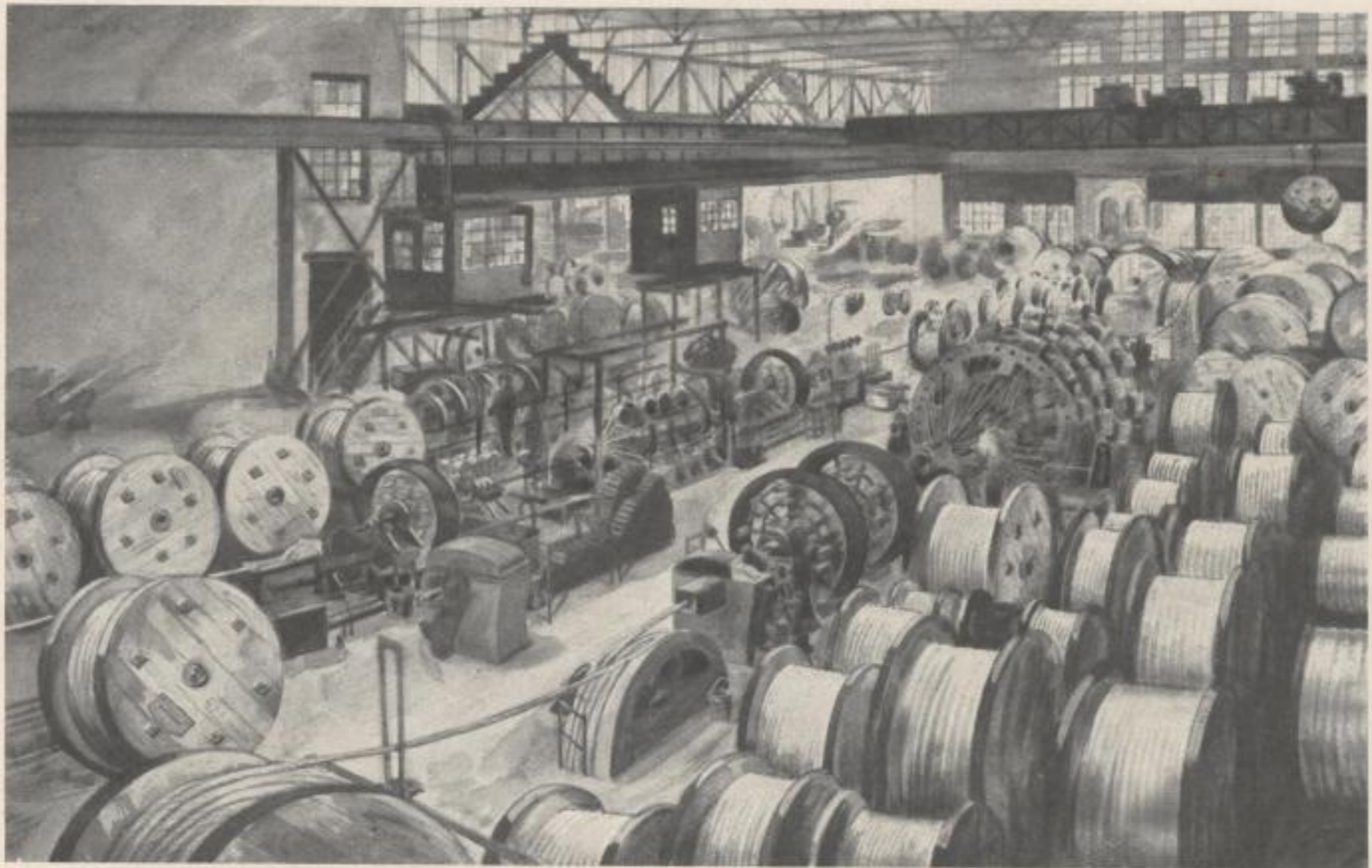
Schwachstrom-Kabelfabrik (Umspinnmaschinen) / Wealz-Current Cable Factory (Winding Machines)
