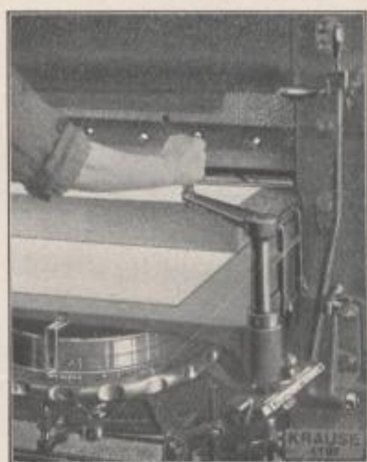
Der haargenau arbeitende und nicht nachlassende mechanische Zahnklinken-Vorschub KRAUSE und die Feineinstellung
