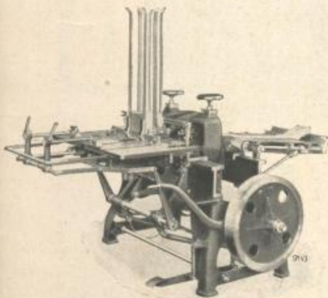
STANZAUTOMAT KRAUSE
