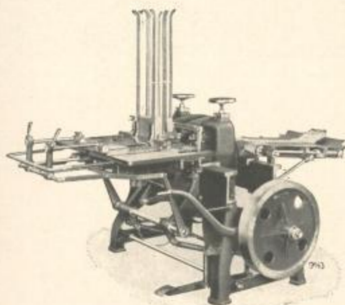
Stanz-Automat
