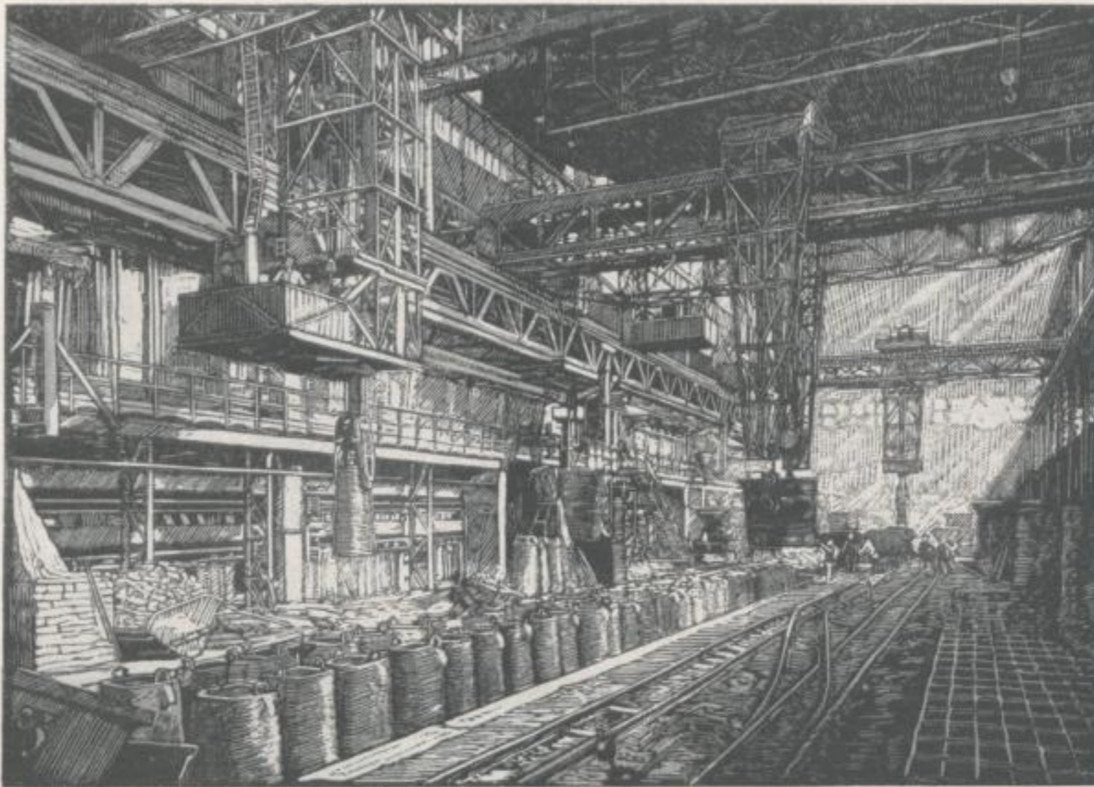
Die Gießhalle eines Martin- stahlwerks Martin Steel-Work
