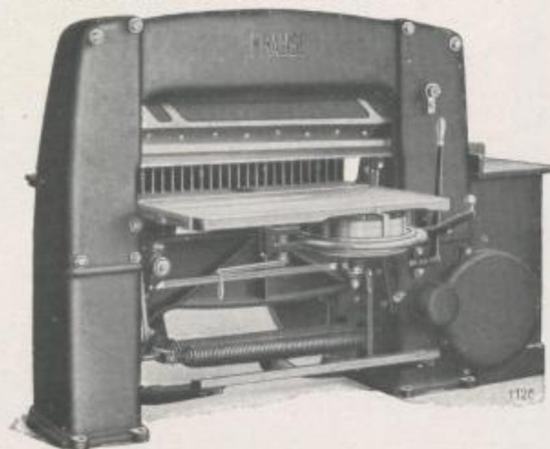
KRAUSE-ULTRA MODELL A-G
