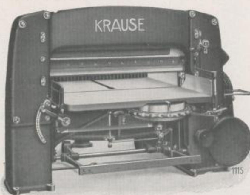
KRAUSE-ULTRA MODELL A-H, A-Hb
