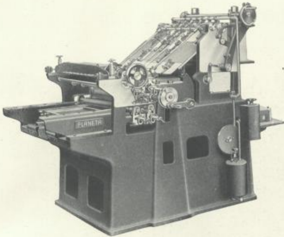
Planeta-Zylinderautomat Dresden-Leipziger Schnellpressenfabrik A.G., Coswig
