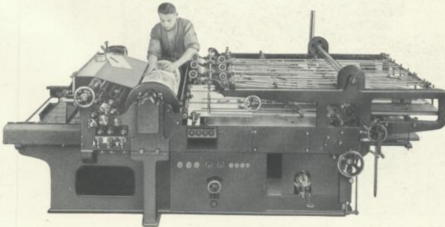
Victoria-Front in Zurichtstellung. Rockstroh, Heidenau
