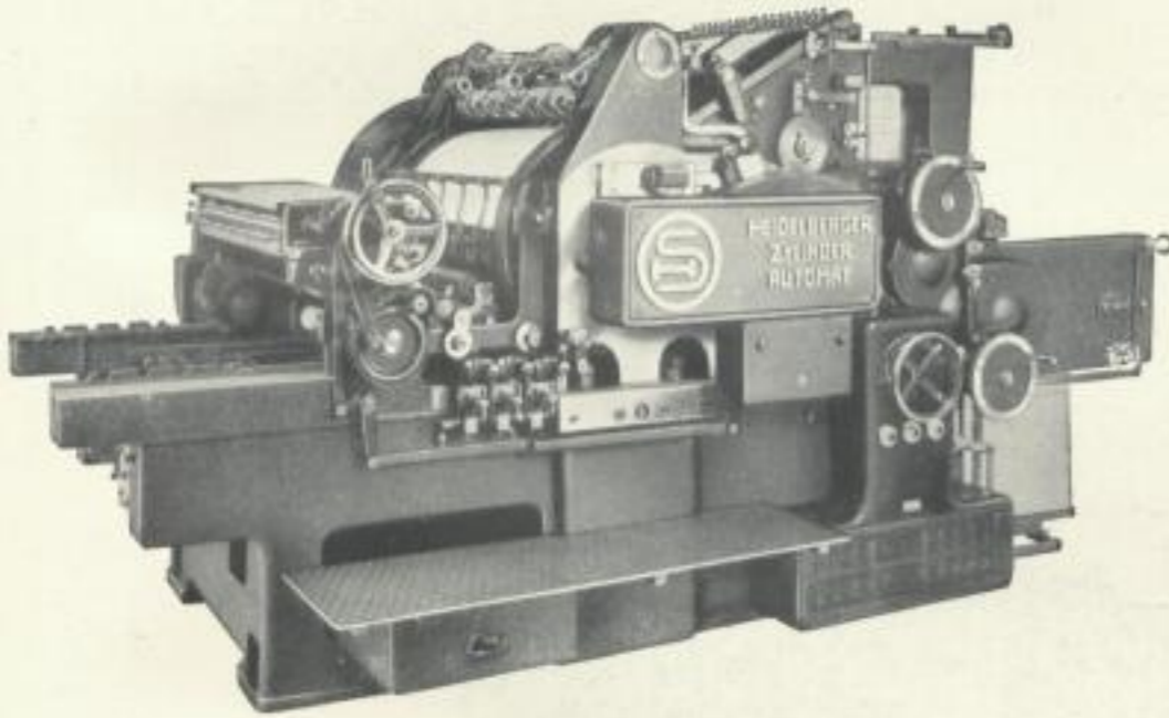
Heidelberger-Zylinder-Automat. Schnellpressenfabrik AG., Heidelberg
