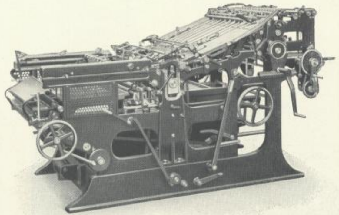
Gesamtansicht vom „Pionier“, Kamenzer Maschinenfabrik Gebr. Heidsieck
