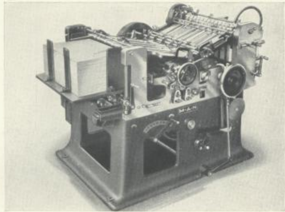
Zweitouren-Automat „Poly“, MAN
