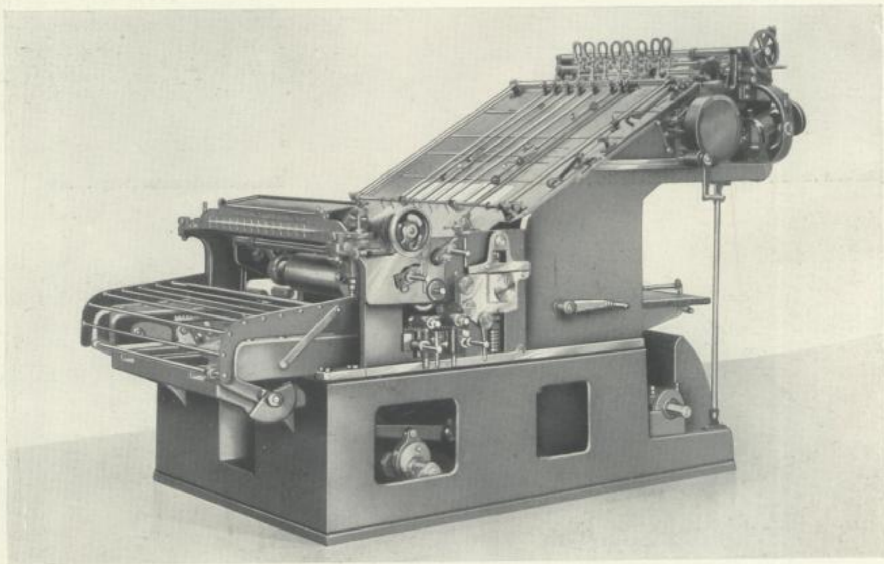
Gesamtansicht vom „Stürmer“. Maschinenfabrik Johannisberg, Geisenheim am Rhein
