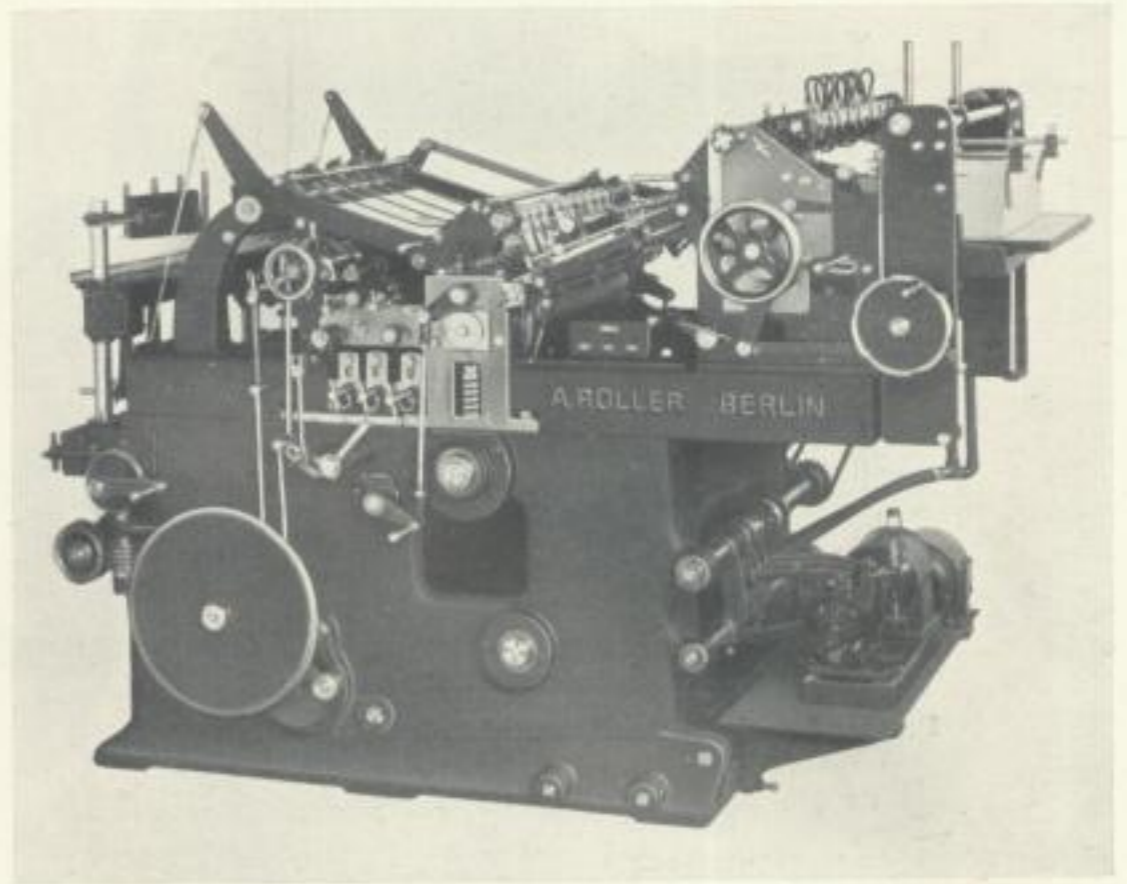
„Roller“. Schwingzylindermaschine mit Frontbogensausgang. A. Roller, Berlin
