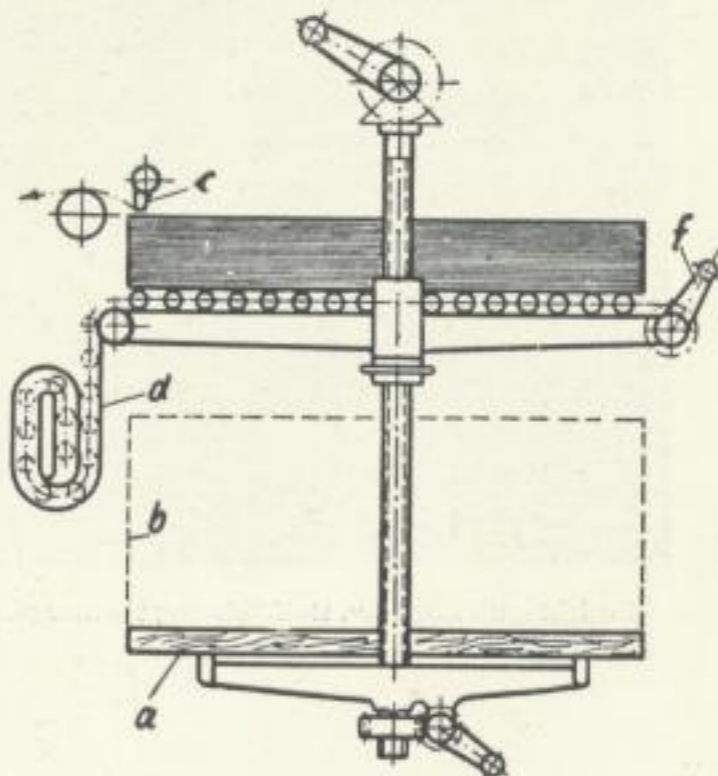
Rolltisch. Koenig-Werk, Berlin
