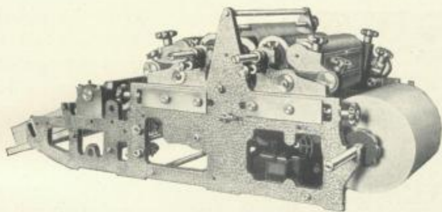
Kleine Kohlbach-Anilindruckmaschine AS. Kohlbach & Co., Leipzig
