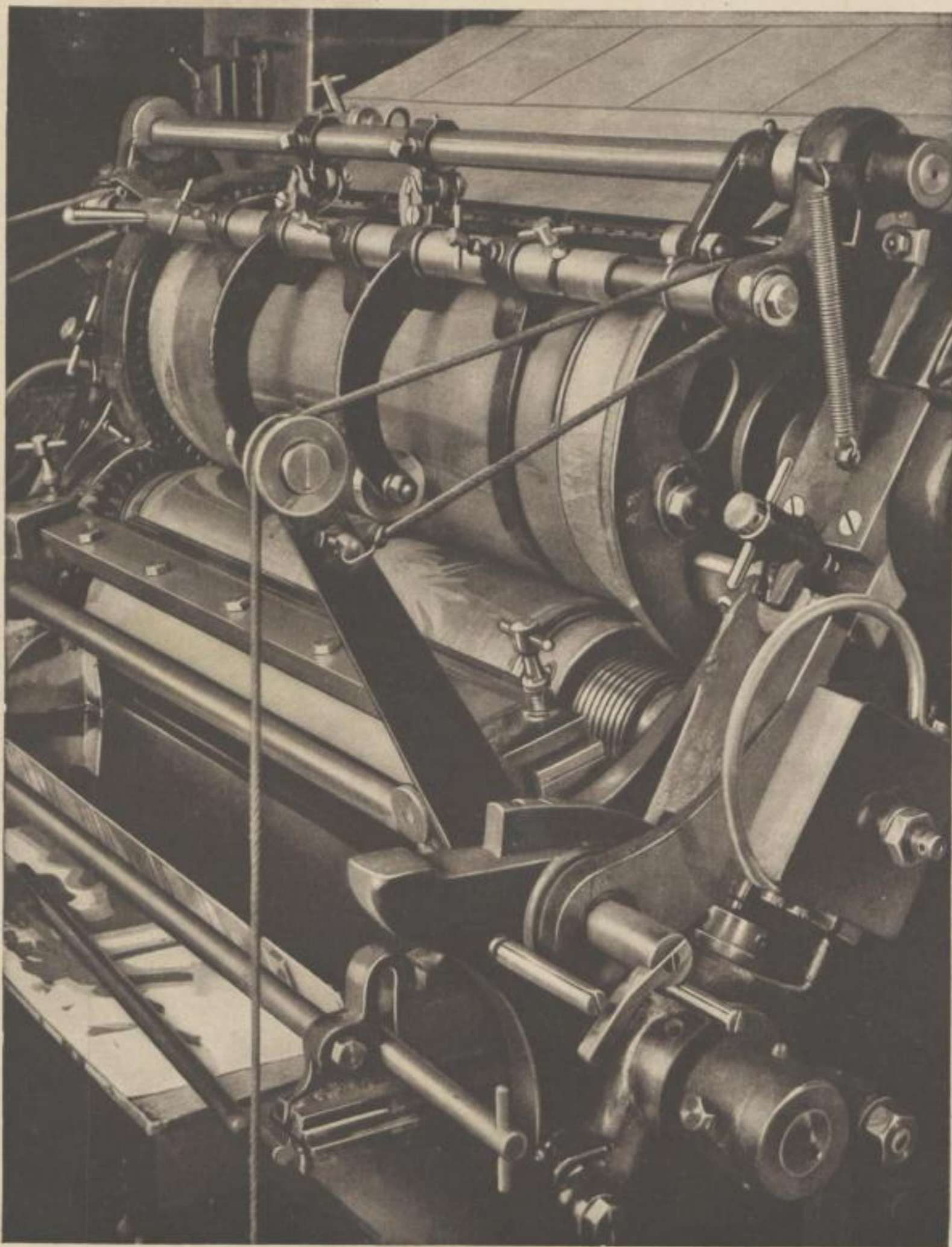
Liti-Tiefdruckmaschine
