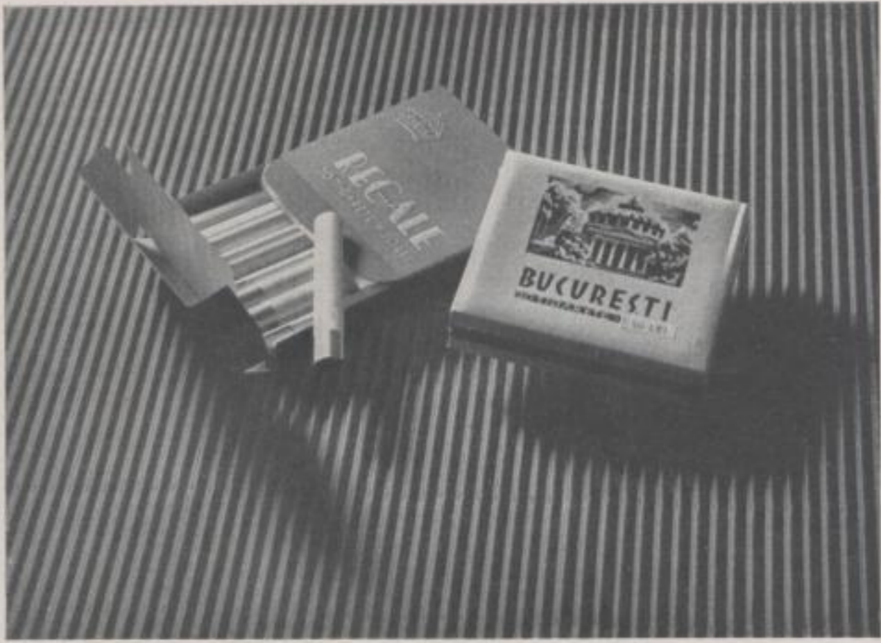
Zigarettenpackungen
