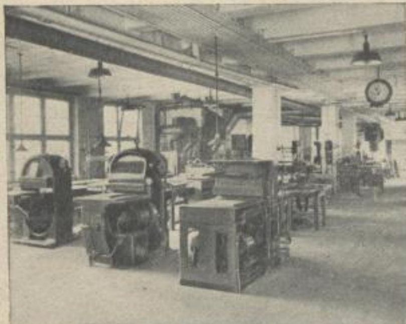
Prägepressen für die Herstellung der Zeitungsmaschinen der MNN
