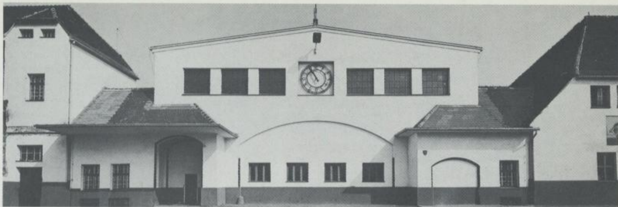
Schlachthof Ostragehege, Giebelansicht Kopfbau der Verbindungshalle, Foto: Kukula 1994
