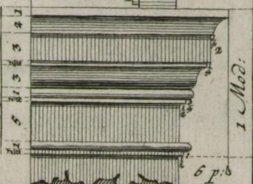
Corinthischer Kämpfer u. Schwibbogen. Römischer Kämpfer und Schwibbogen.
