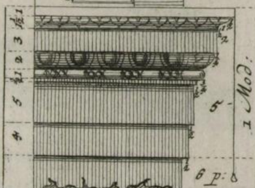
Dorischer Kämpfer und Schwibbogen Ionischer Kämpfer u. Schwibbogen.
