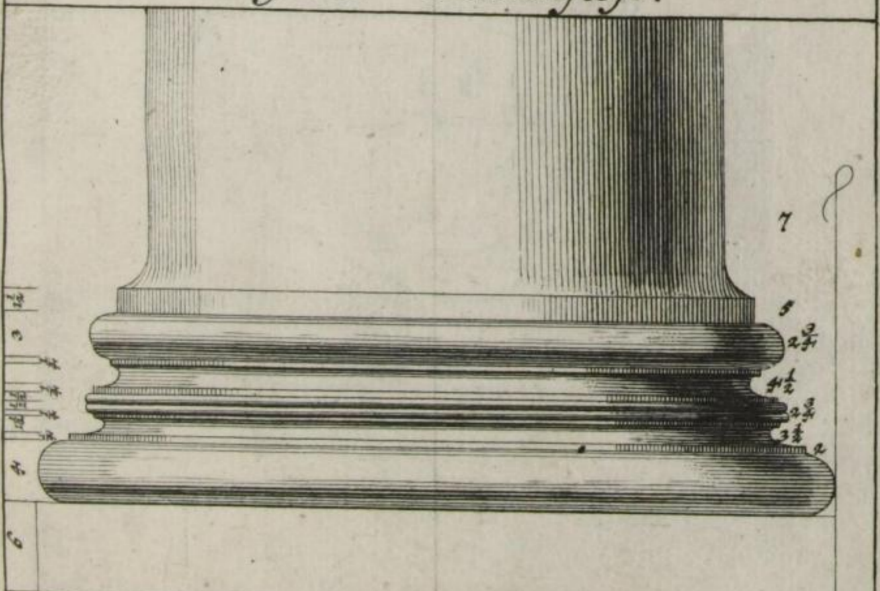
Corinthischer Säulenfuß.
