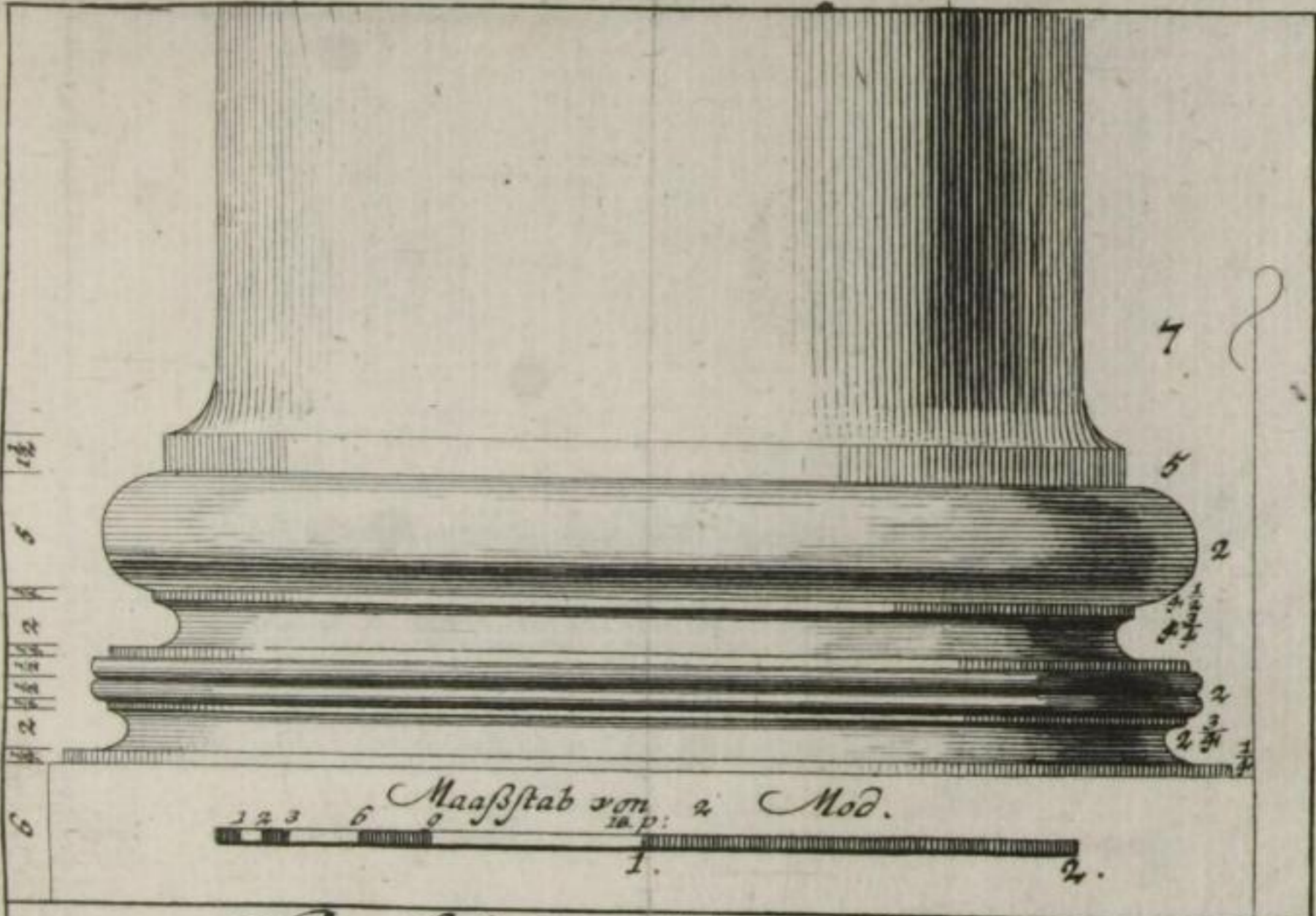
Ionischer Säulenfuß.
