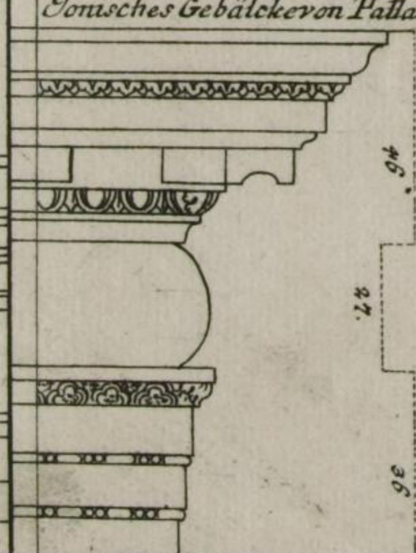
Alte und Neue Ionische Gebälcke. 50.
