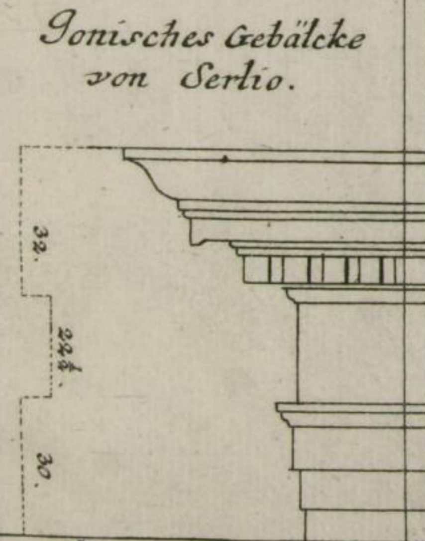
Alte und Neue Ionische Gebälcke. 50.
