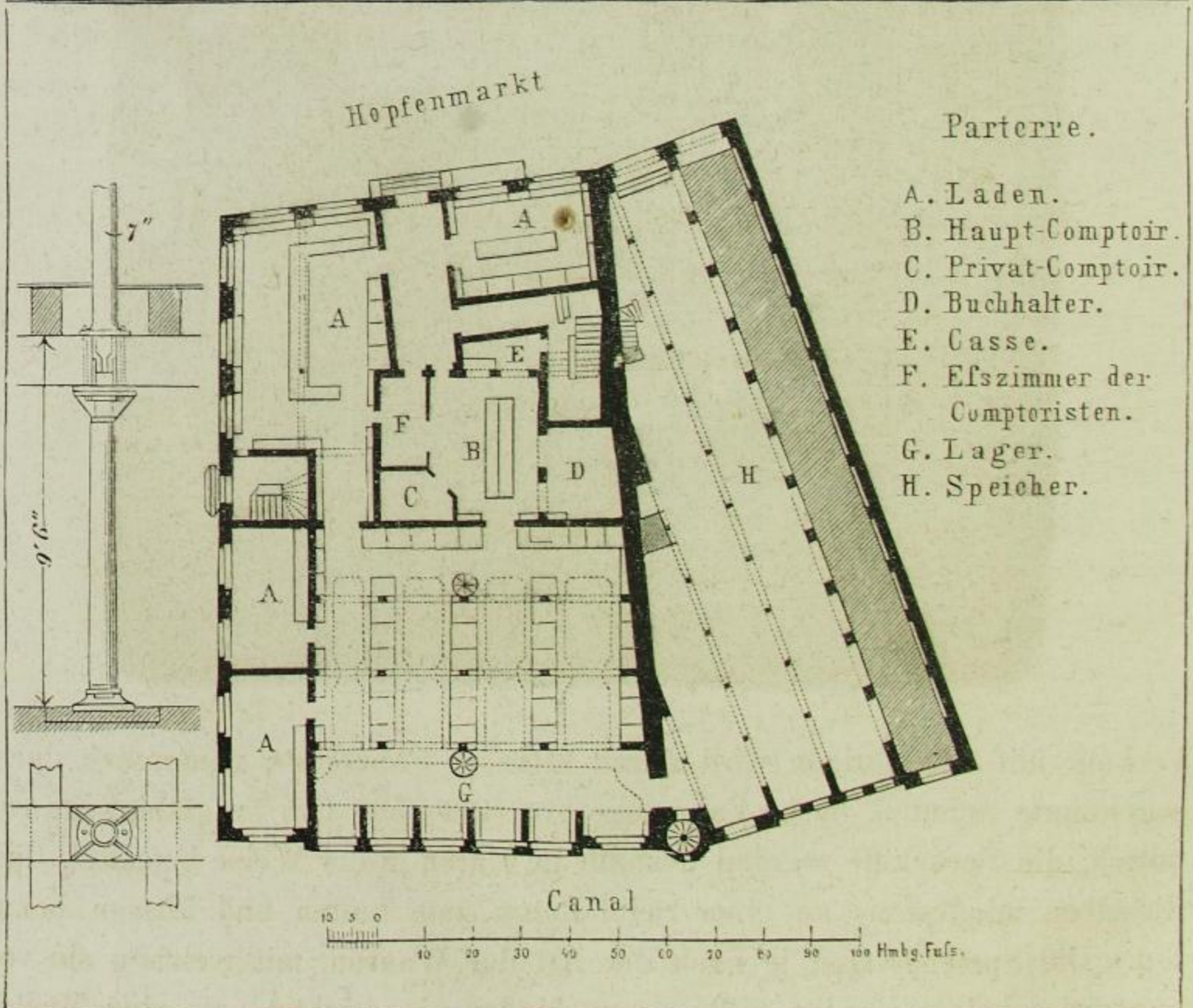
Speicher von Schulte & Schemmann.
