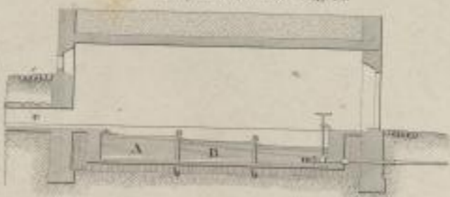
Längenschnitt
