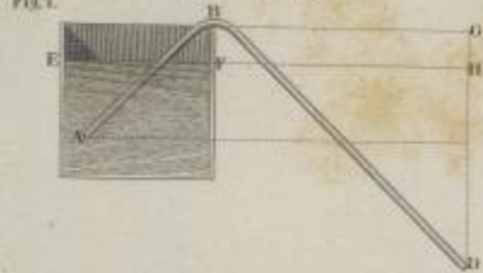
Heber am Kanal von Languedoc. Längsprofil durch den Kanal.
