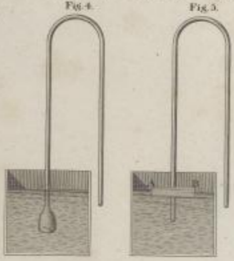
Ventilheber. Heber mit Schwimmer. Diabolo.
