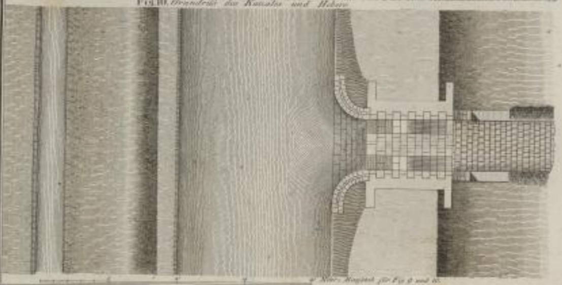
Fig. 10. Grundriß des Kanals und Hebers.
