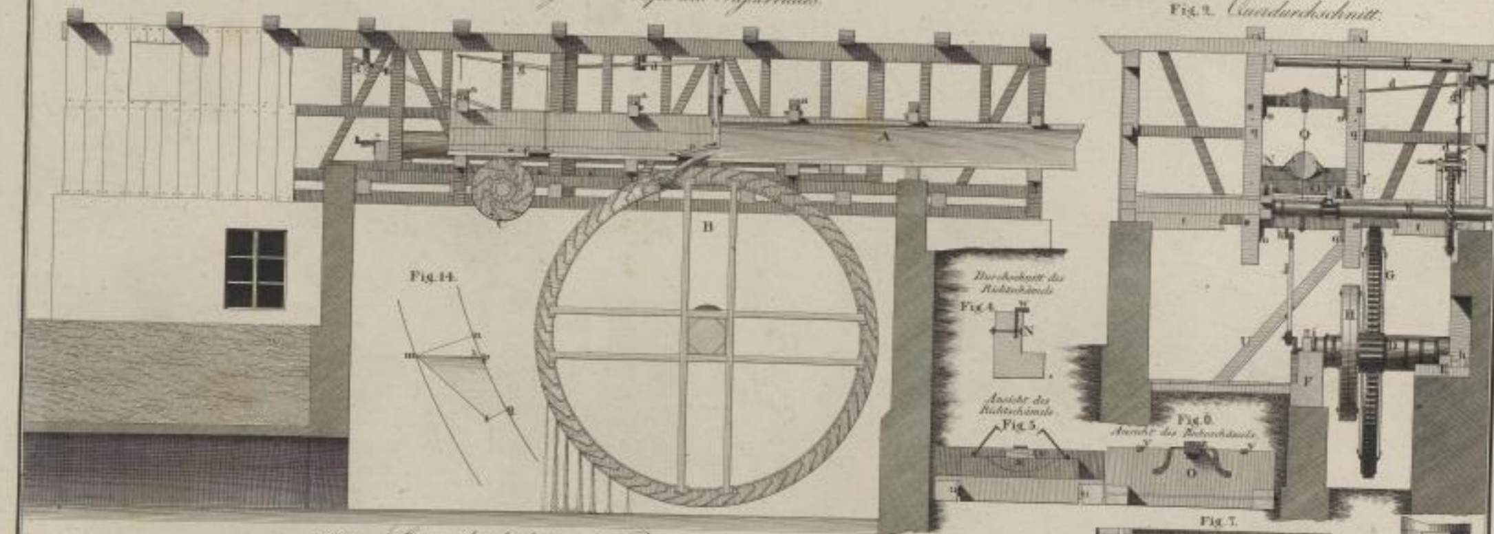
Fig. 3. Längendurchschnitt der Bretsäge.
