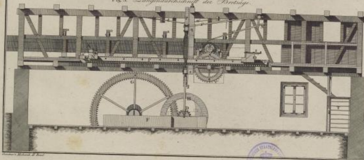
Fig. 3. Längendurchschnitt der Bretsäge.
