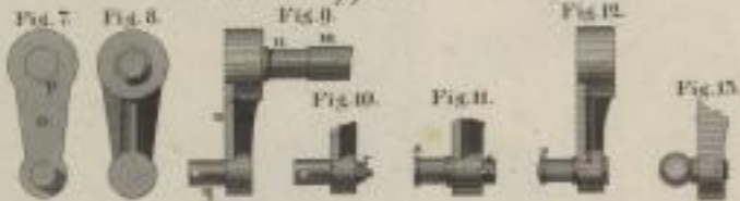
Offene Zapfenlager.
