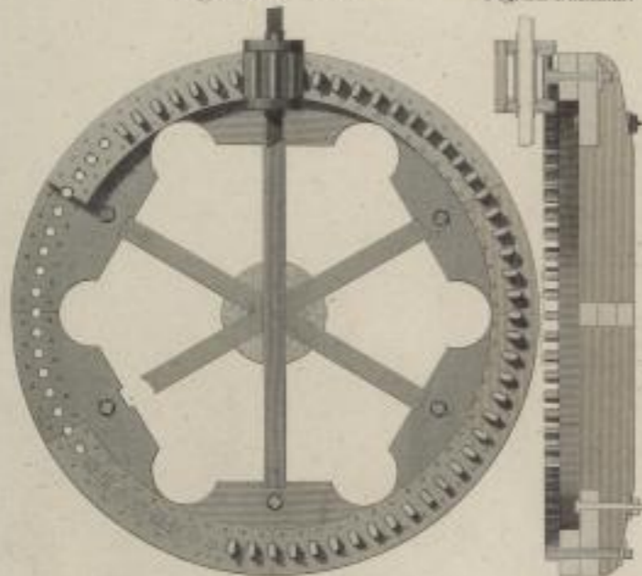
Fig. 1. Vorder Ansicht
