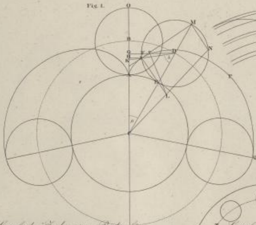
Gestalt der Zähne eines Rades für das Beispiel, Seite 39, Band III.
