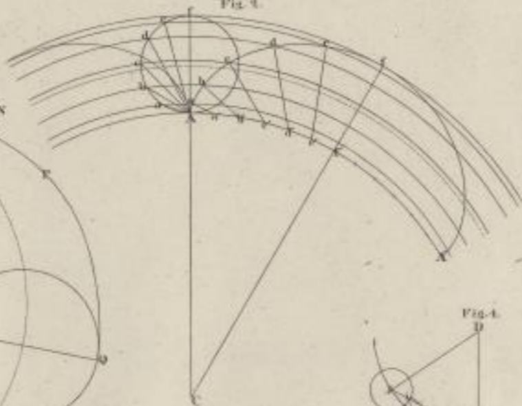
Vervollständigung des Epicycloids.
