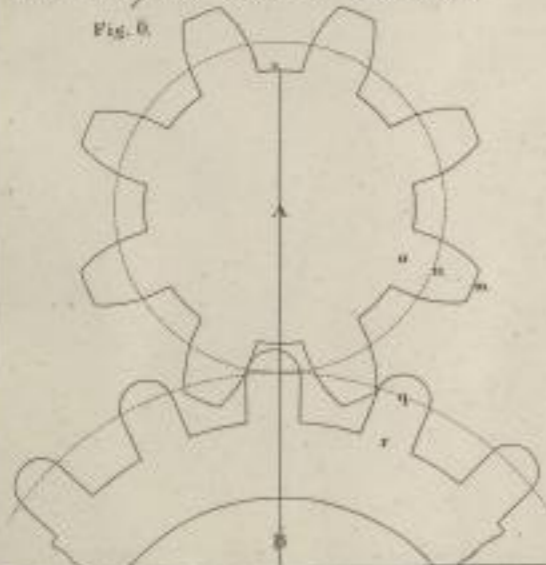
Gestalt der Zähne eines Rades für das Beispiel, Seite 39, Band III.
