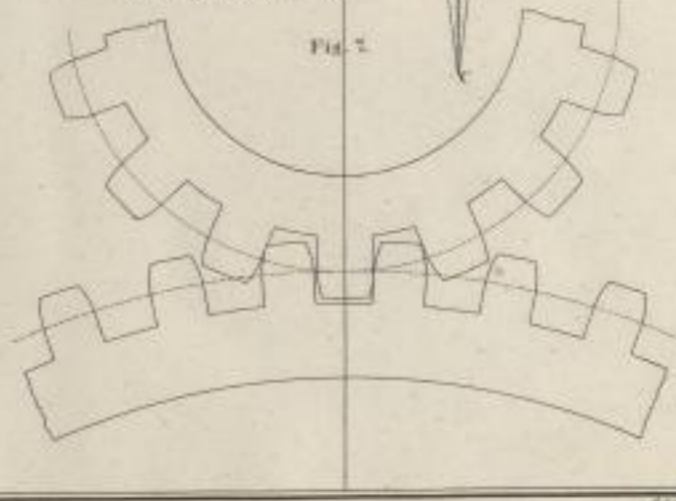
Gestalt der Zähne metallener Räder für das Beispiel, Seite 40, Band III.
