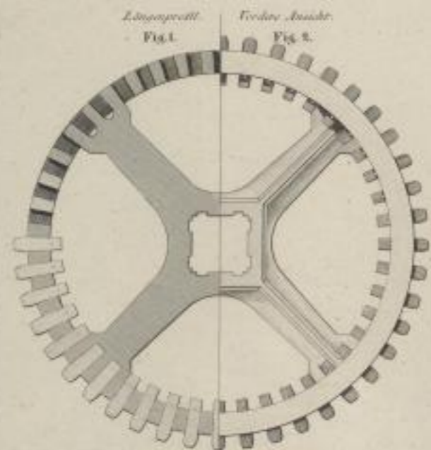
Rad mit gusseisernem Kranze und hölzernen Zähnen.
