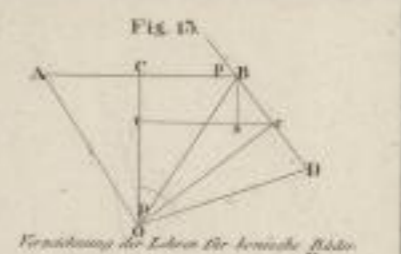
Bildung konischer Räder.
