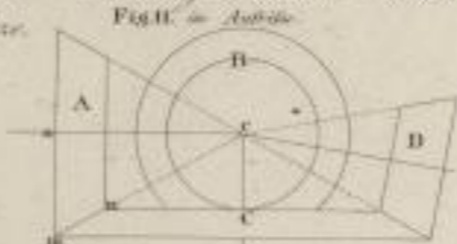
Bildung konischer Räder.
