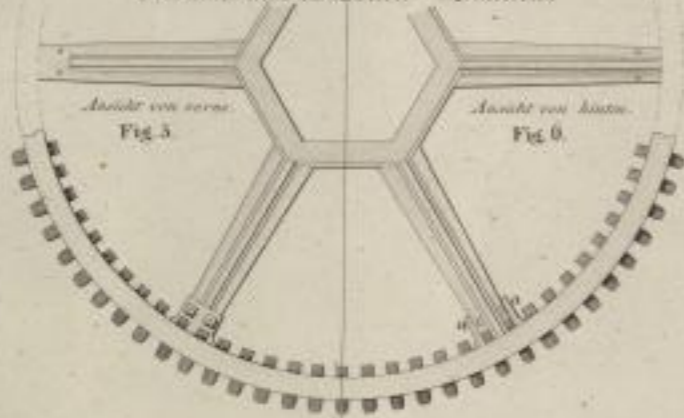
Rad mit gusseisernem, an die Arme angeschraubtem Kranze und hölzernen Zähnen.
