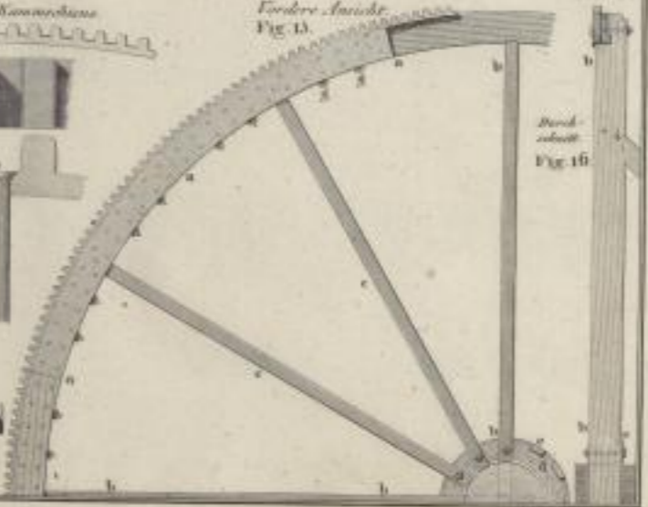
Keilernes Rad mit eisernen Nüssen.
