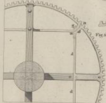
Fig. 14. Durchschnitt des Rades.
