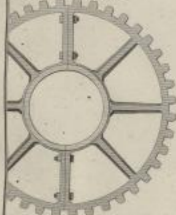
Fig. 10. Durchschnitt des Rades.
