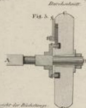
Lose Rolle mit einem gegen das feste Kuppelungsstück vorgesteckten Ringel
