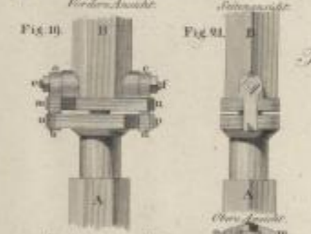
Kuppelung mittelst beweglicher Arme
