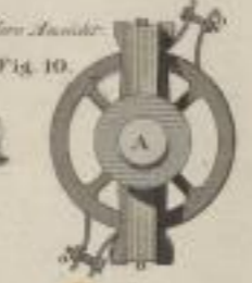
Nachgebende Kuppelung zweier Wellen
