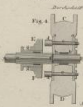
Nachgebende Kuppelung eines Triebrades mit einer Welle
