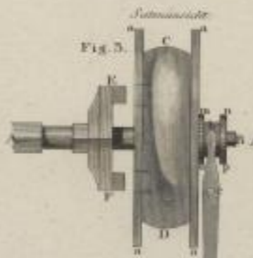
Nachgebende Kuppelung eines Triebrades mit einer Welle
