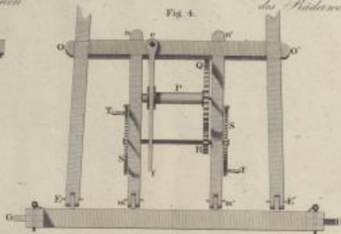
Vordere Ansicht
