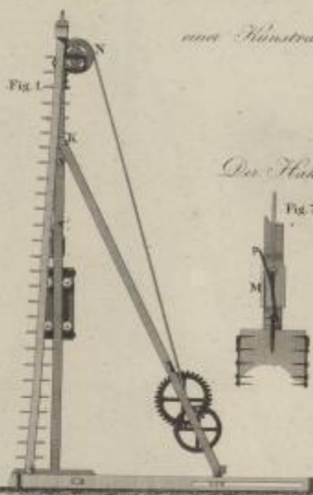
Seitenansicht
