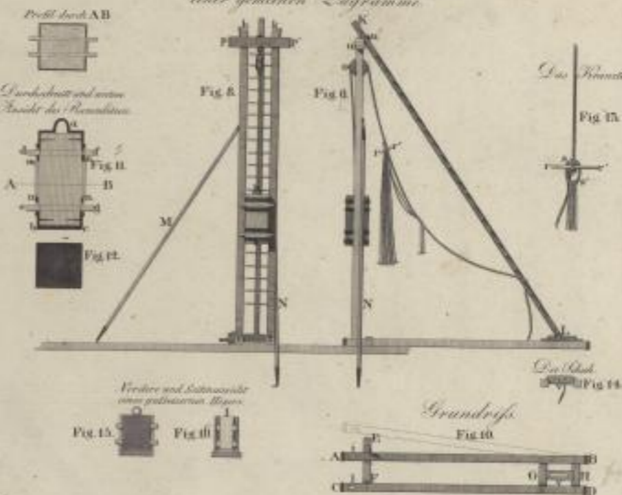
Vordere Ansicht
