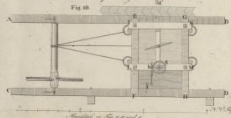
Obere Ansicht der Pflahlsäge
