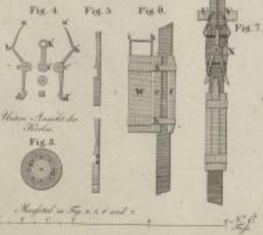
Bestandtheile der Säge
