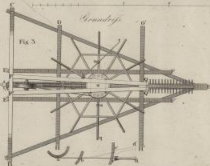
Obere Ansicht der Pflahlsäge
