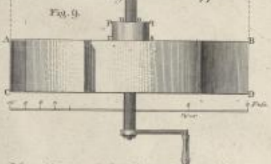
Ansicht einer Spiralmaschine, welche durch ein Wasserrad bewegt wird.
