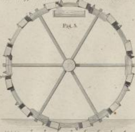
Ansicht eines Schöpfrades mit an der Seite gebrachten Wasserkränzen.
