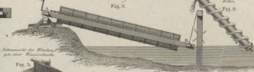
Ansicht einer Wasserschnecke und des bei ihrem Gebrauche nöthigen Gerüsts.
