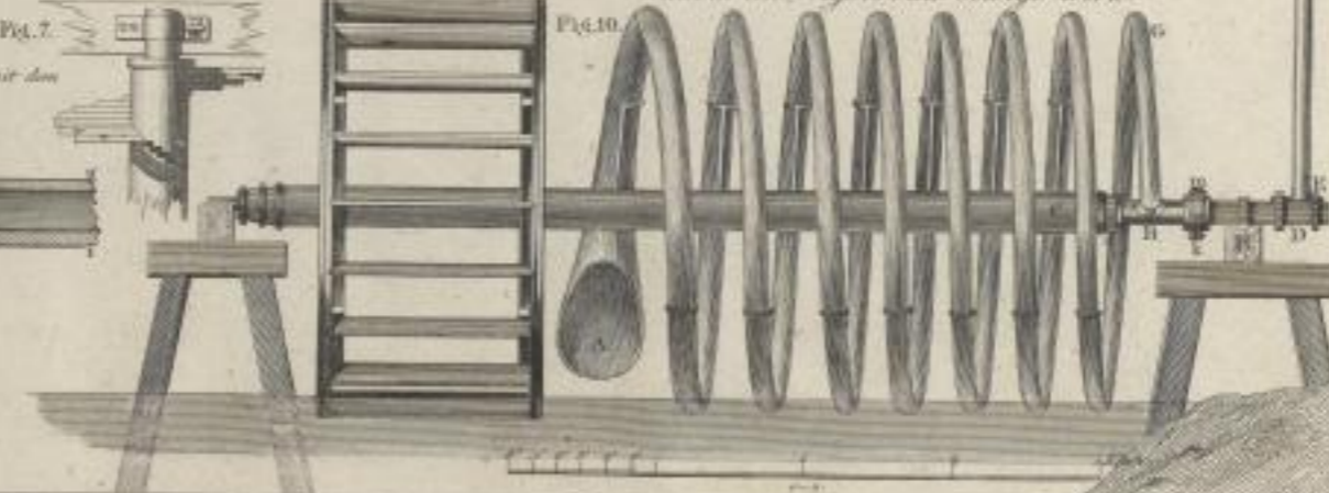
Ansicht einer Spiralmaschine, welche durch ein Wasserrad bewegt wird.
