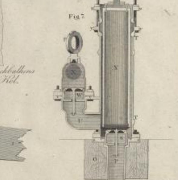
Durchschnitt des Stiefels in Verbindung mit dem Saug- und Abstreicher.
