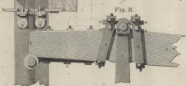
Seitenansicht eines Druckbalkens in Verbindung mit der Rollenstange.
