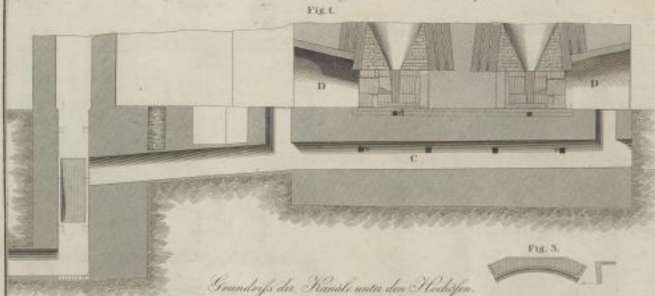
Längendurchschnitt durch die Abzugswälle beider Hochöfen.
