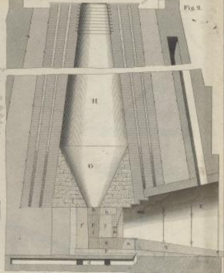
Vordere Ansicht des Abzugswalles.
