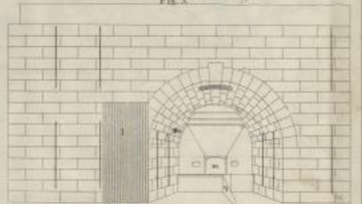
Vordere Ansicht des Abzugswalles.
