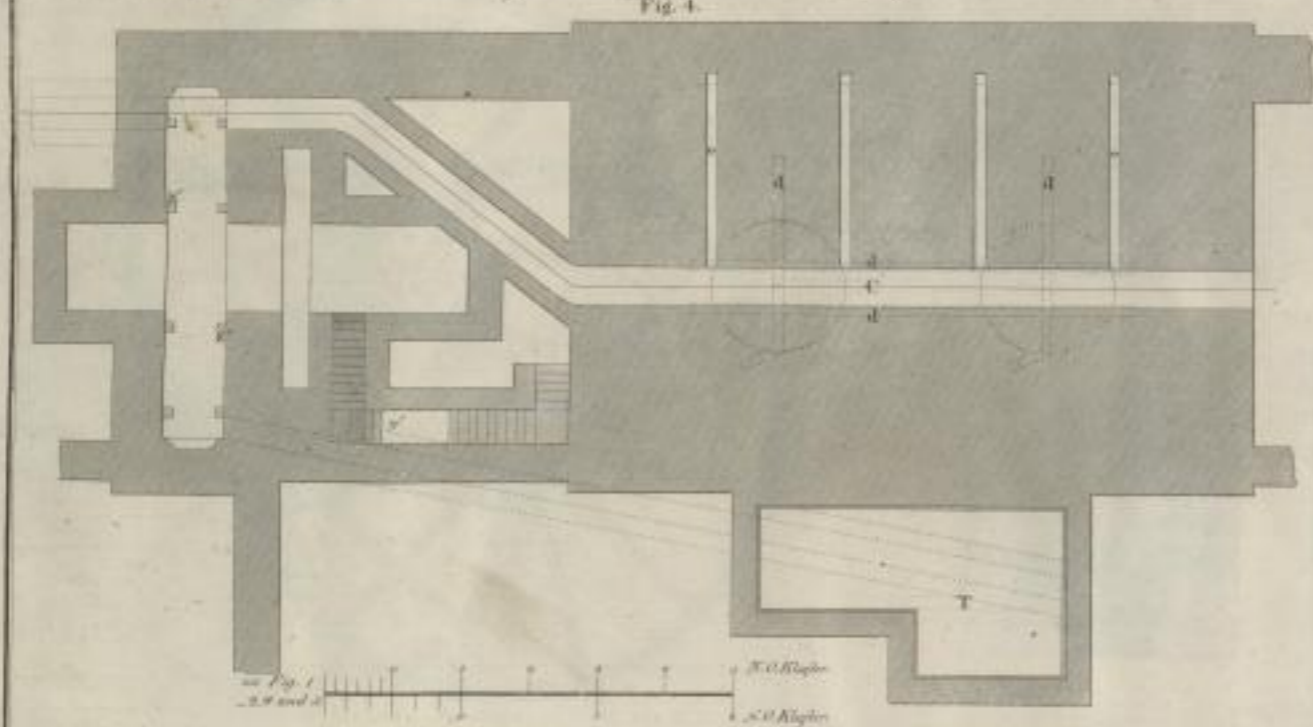
Grundriß des Kanals unter den Hochöfen.
