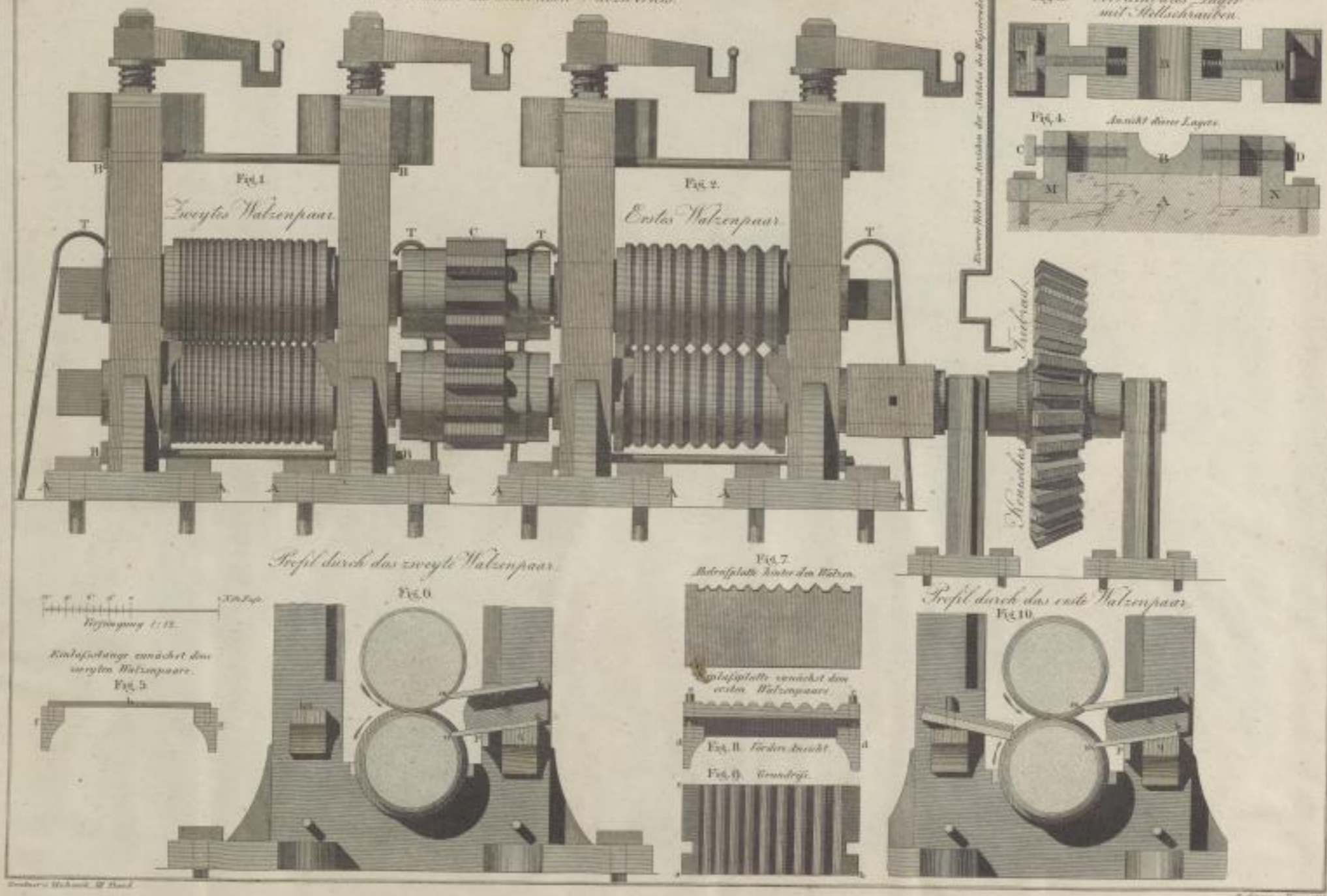
Vordere Ansicht des Stabeisen-Walzwerks.
