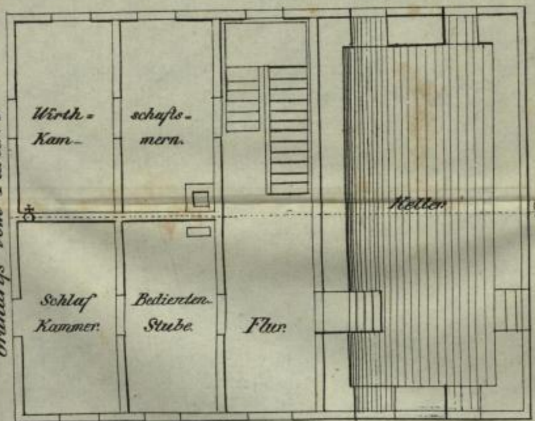
Grundriß vom Parterre.
