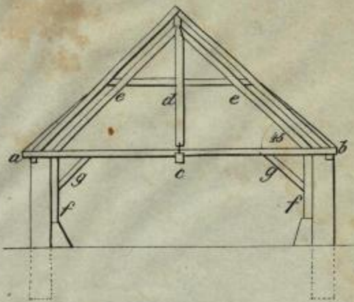
Profil eines Hangwerk-Binders im Schafstall.
