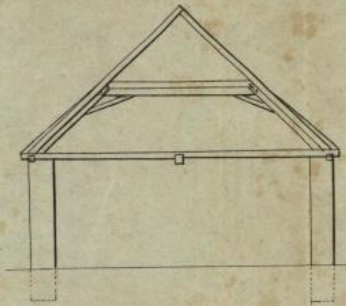
Profil eines Dach-Binders im Schafstall.
