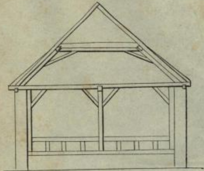
Profil eines Dach-Binders in der Scheune.
