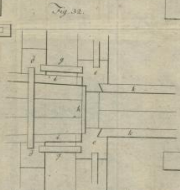
Grund und Aufsicht der Zimmerung vor der Schürze
