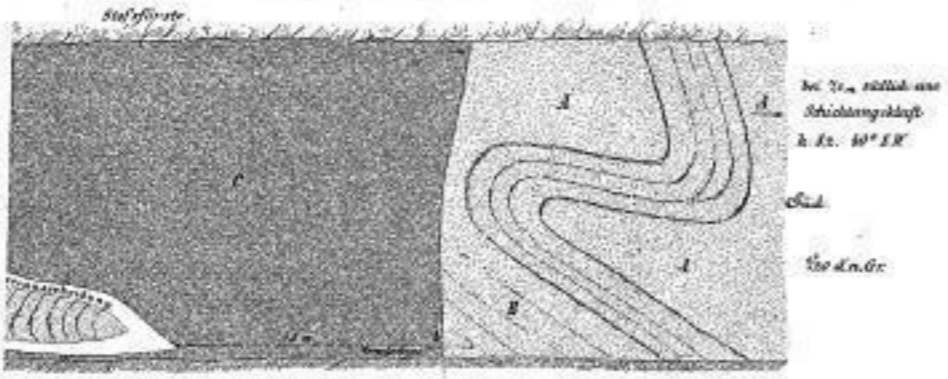
Fig. 2. Skizze Metallwerkstätte im Fürstenbau über 6. Gangstrecke a. 2. Silberfund Stahenden 50m v. Neuglück Spat in Nord. Aufgenommen am 10. August 1870. Ansicht der östlichen Wand.
