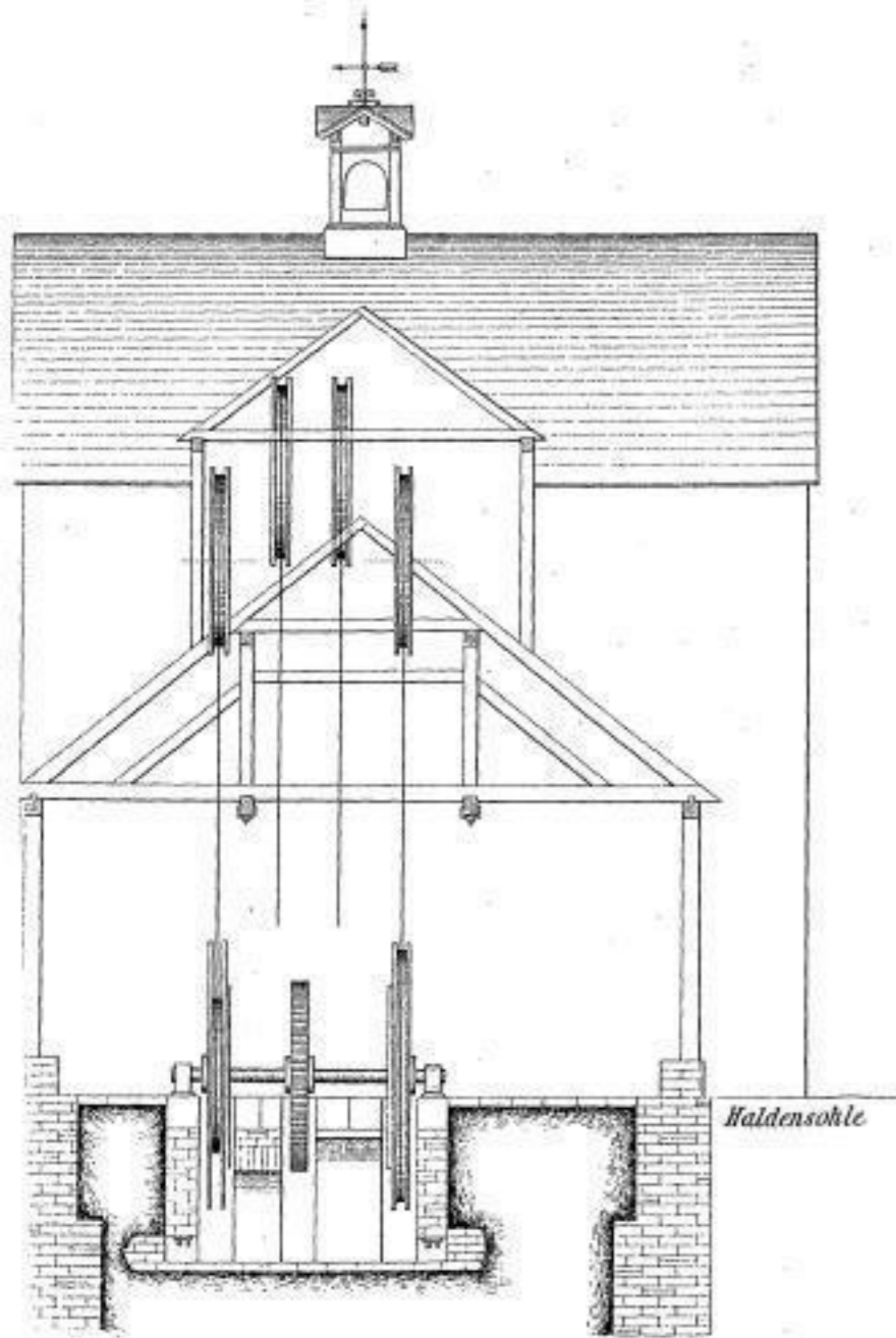
Fig. 1 Querschnitt.
