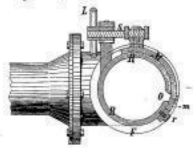
Fig. 3. Schnitt A B.
