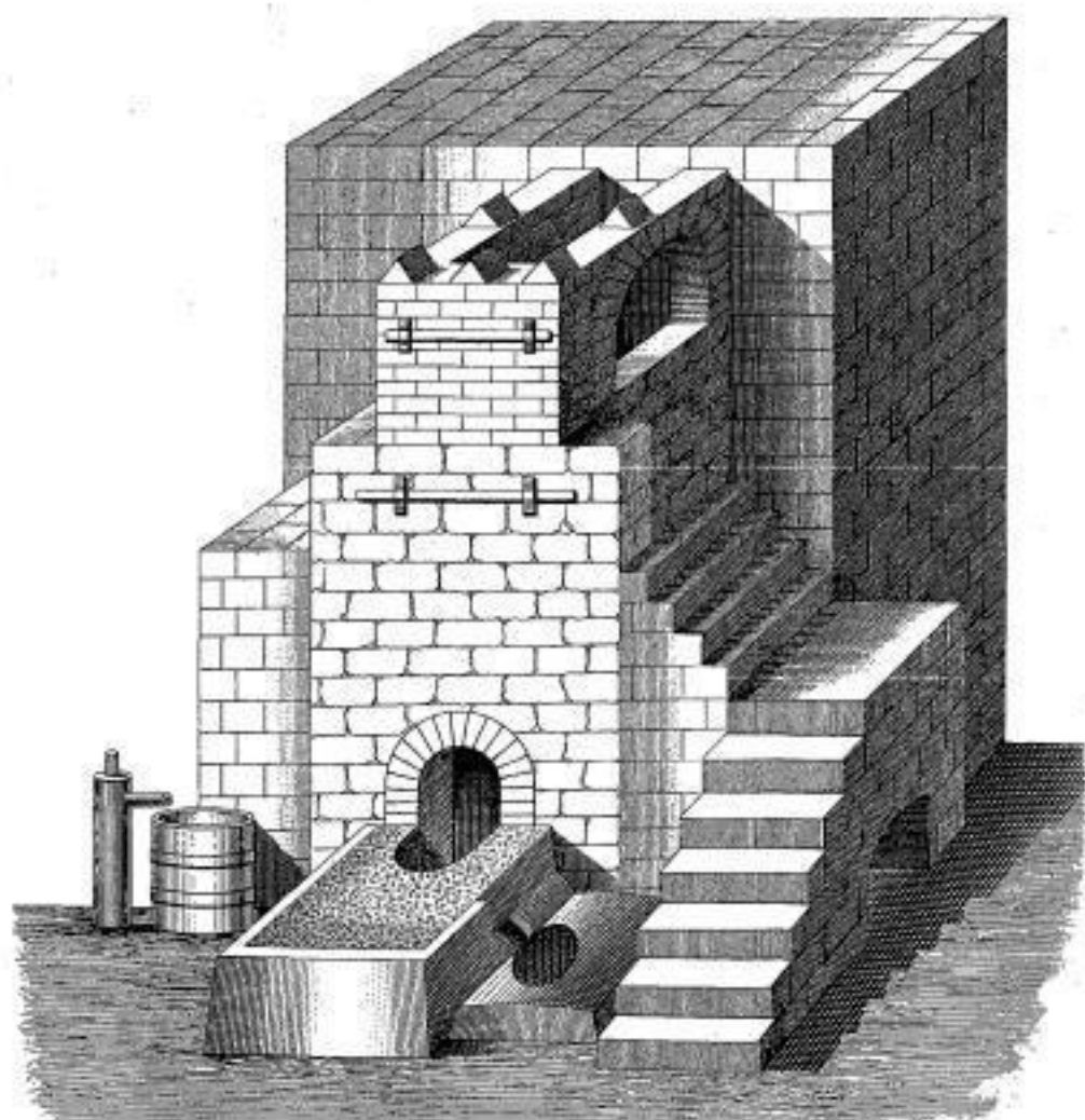
Freiberger Schachtöfen aus dem 18. Jahrhundert.
