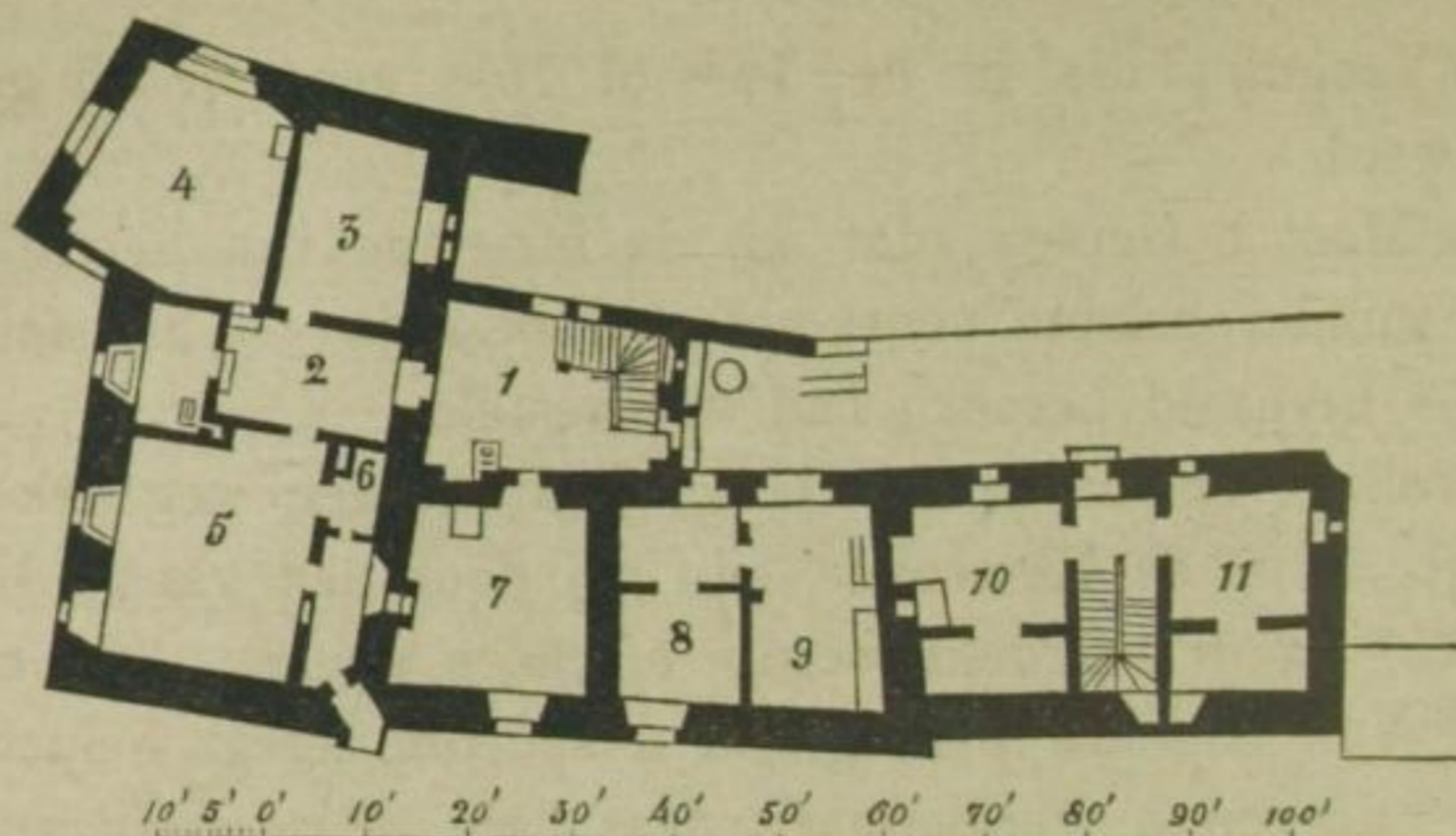
Plattegrond der benedenverdieping van het Ridderhuis.
