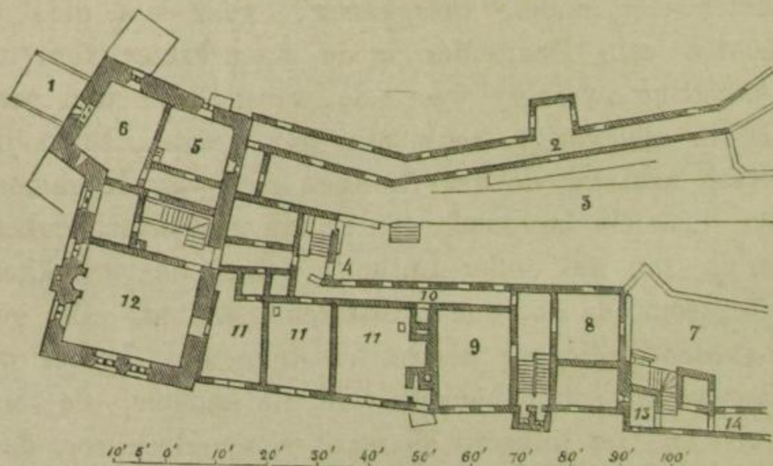
Plattegrond der tweede verdieping van het Ridderhuis.
