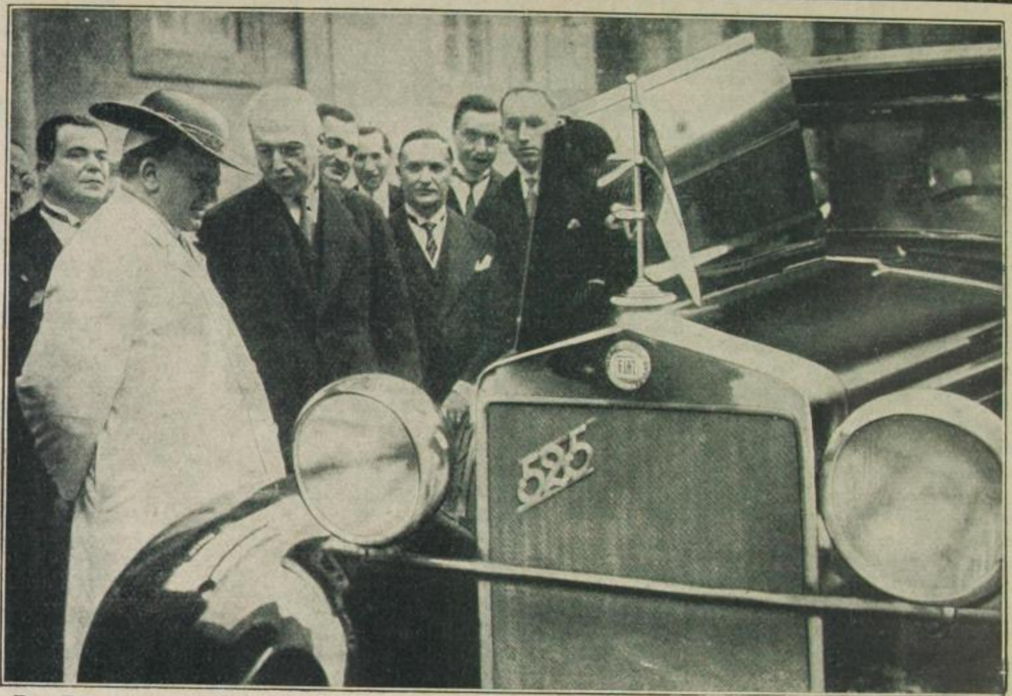
„Der Präsident der Fiat-Werke, Senator Agnelli, erklärt vor dem Vatikan dem Papst Einzelheiten am Motor des neuen 15/70 PS Fiat Modell 525, der ihm von der Fiat geschenkt wurde.“
