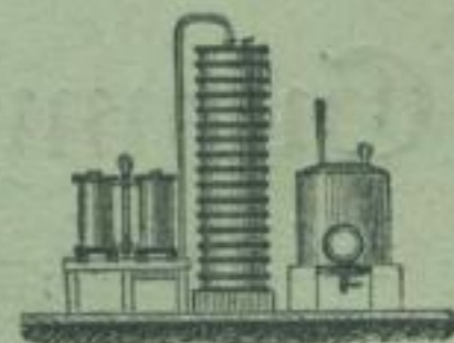
Ammoniak-Apparat.
