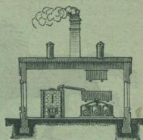
Destillations-Anlage.
