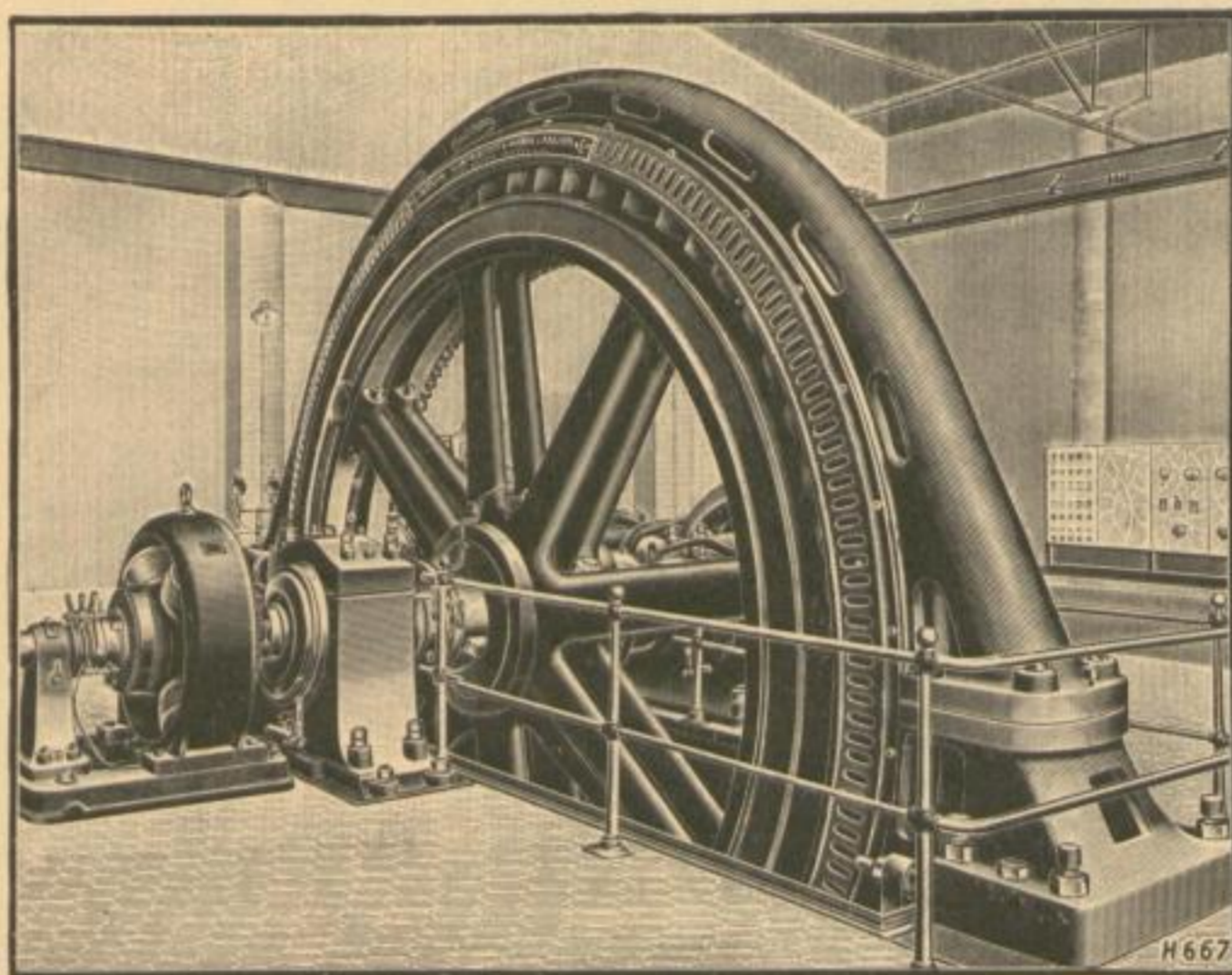
Drehstrom-Generator, Modell NJ 107/105, 500 Volt, 500 KVA, 107 Umdrehungen in der Minute, 50 Perioden, mit einem GD^2 = \text{ca. } 400000 \text{ kgm}^2 .
