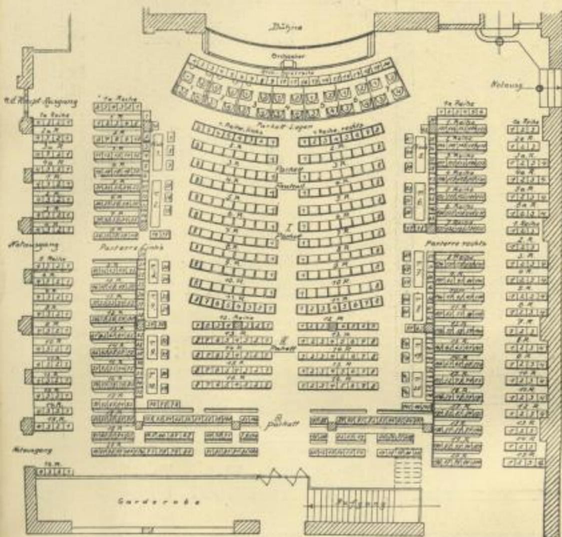
Grundriß vom Erdgeschoss
