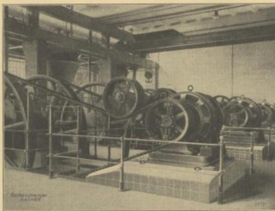
Brikettpressenantrieb durch Drehstrommotoren 5000 Volt, 180 KW, 50 Per., 490 Umdrehungen p. Minute
