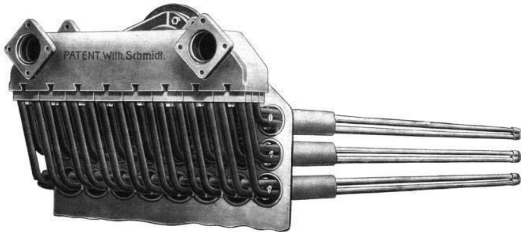
Fig. 15. Rauchröhren-Überhitzer, Pat. Wilh. Schmidt.
